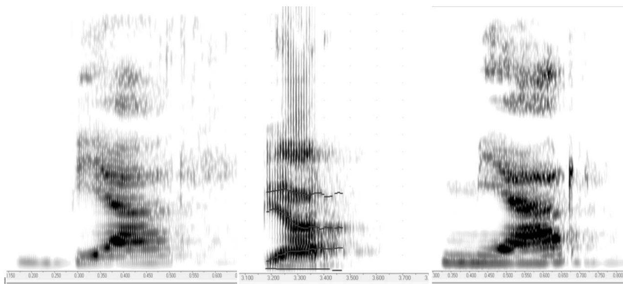
Фигура 2. Спектрограми на б'ар , п'ар , м'ар в българския език
