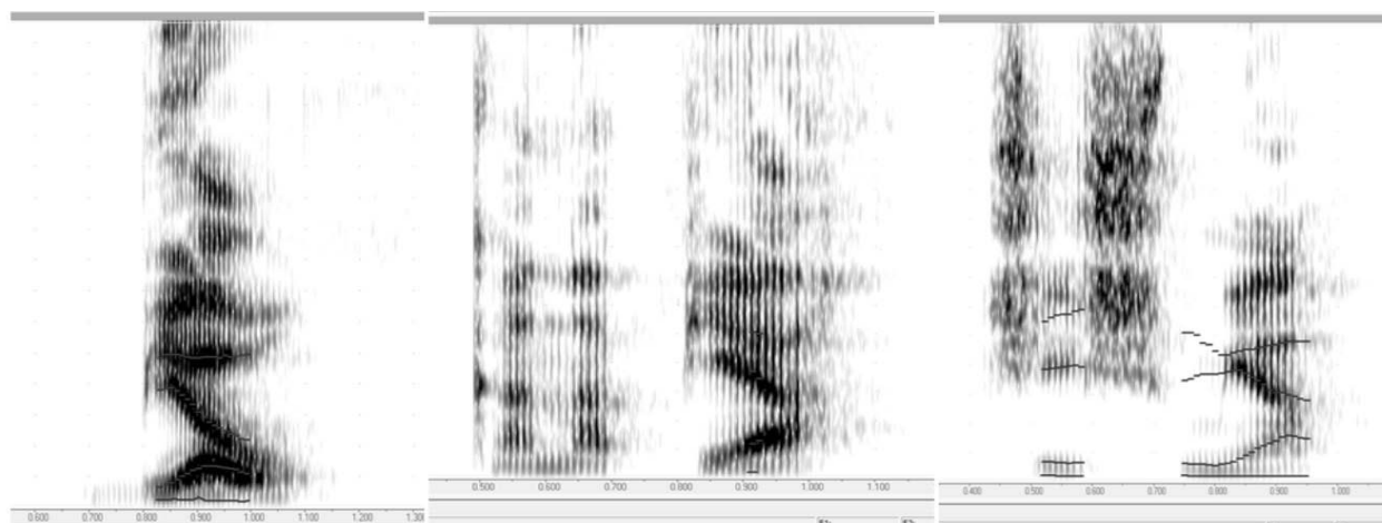
Фигура 3. Спектрограми на beau 'пия', canapea 'канapé' и ciștea 'чешма' в румънския език
